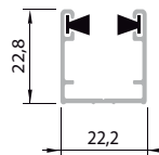
Guía inferior/ Inferior guide/ Inferior Coulissee CÓDIGO BLANCO - 90070124 CODE FOR WHITE. CODE POUR BLANC.
