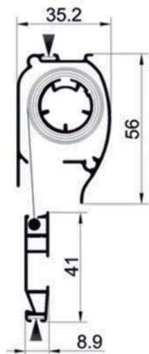
Cabezal 35/Caisson 35/Box 35 CÓDIGO BLANCO - 90070011 ( tela/toile/mesh 180) CODE FOR WHITE. CODE POUR BLANC.
