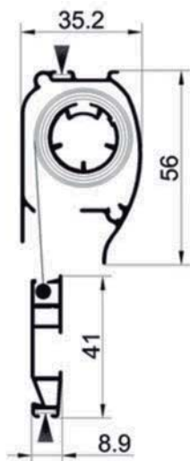
Cabezal 35/Caisson 35/Box 35 CÓDIGO BLANCO - 90070011 ( tela/toile/mesh 180) CODE FOR WHITE. CODE POUR BLANC.
