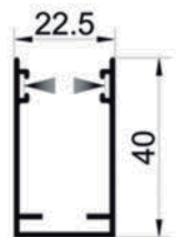
Guía /Guide/Guide CÓDIGO BLANCO - 90070033 CODE FOR WHITE. CODE POUR BLANC.
