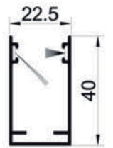
Guía Antiviento/ Guide windproof/ Coulissee Anti-vent CÓDIGO BLANCO - 90070042 CODE FOR WHITE. CODE POUR BLANC.
