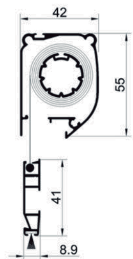
Cabezal 42/Caisson 42/Box 42 CÓDIGO BLANCO - 90070070 ( tela/toile/mesh 240) 90070079 (tela/toile/ mesh 180) CODE FOR WHITE. CODE POUR BLANC.
