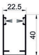
Guía /Guide/Guide CÓDIGO BLANCO - 90070033 CODE FOR WHITE. CODE POUR BLANC.
