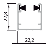
Guía Antiviento/ Guide windproof/ Coulisse Anti-vent CÓDIGO BLANCO - 90070042 CODE FOR WHITE. CODE POUR BLANC.
