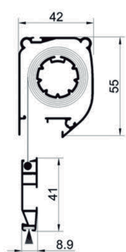
Cabezal 42/Caisson 42/Box 42 CÓDIGO BLANCO - 90070070 ( tela/toile/ mesh 240) 90070079 (tela/toile/ mesh 180) CODE FOR WHITE. CODE POUR BLANC.
