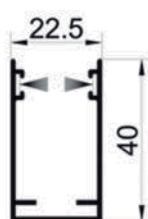
Guía /Guide/ Guide CÓDIGO BLANCO - 90070033 CODE FOR WHITE. CODE POUR BLANC.
