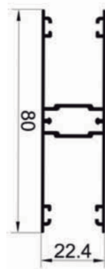
Guía doble/ Double guide/ Double Guide CÓDIGO BLANCO - 90070110 CODE FOR WHITE. CODE POUR BLANC.
