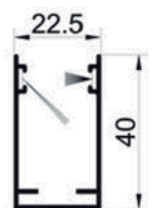
Guía Antiviento/ Guide windproof/ Coulisse Anti-vent CÓDIGO BLANCO - 90070042 CODE FOR WHITE. CODE POUR BLANC.
